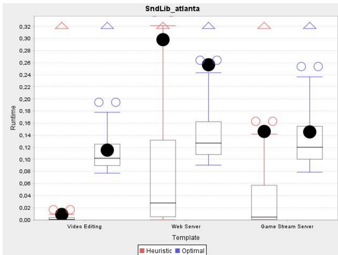
Παράδειγμα BoxPlot
