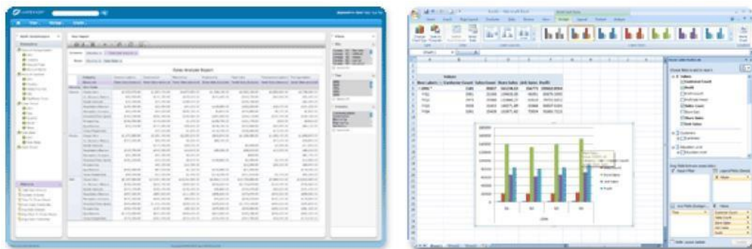
Σχήμα 2-3: OLAP
