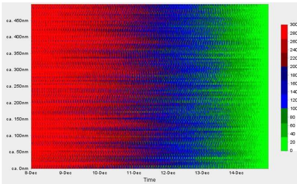
Παράδειγμα HeatMap
